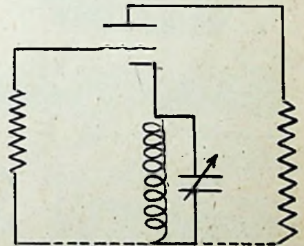
Aequivalent van het gebruikte oscillatorcircuit voor additieve detectie
