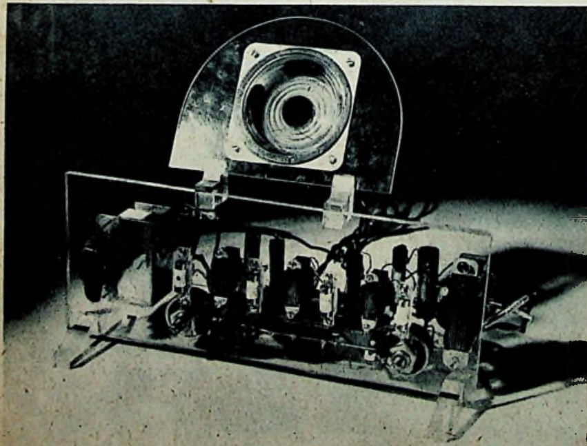
Het eerste complete ontvangtoestel met germanium-kristaltrioden en dioden uitgerust, afkomstig van Westinghouse (Research-afdeling, Parijs)
