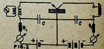
Principeschema van een kristaltriode. Waarden voor de beveiligingsweerstand R_1 en R_2 resp. 500 à 1000 en 10.000 à 20.000 ohm. R_3 is de belastingsweerstand
