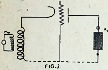
Buisaequivalent van het gegeven prinsipeschema. R_1 = belastingsweerstand
