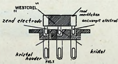
Westcrel-kristal met houder
