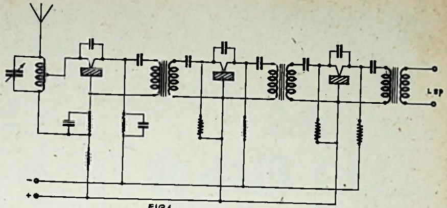
Prinsipeschema van de eerste Westinghouse kristaltriode-omroepontvanger
